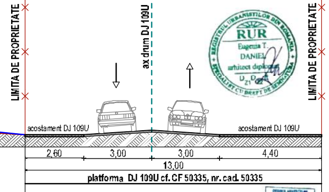
PROFIL TRANSVERSAL A-
